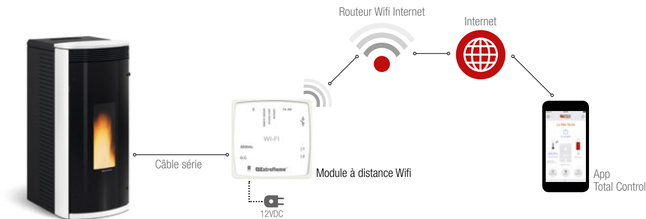
Schéma Module à distance Wifi
