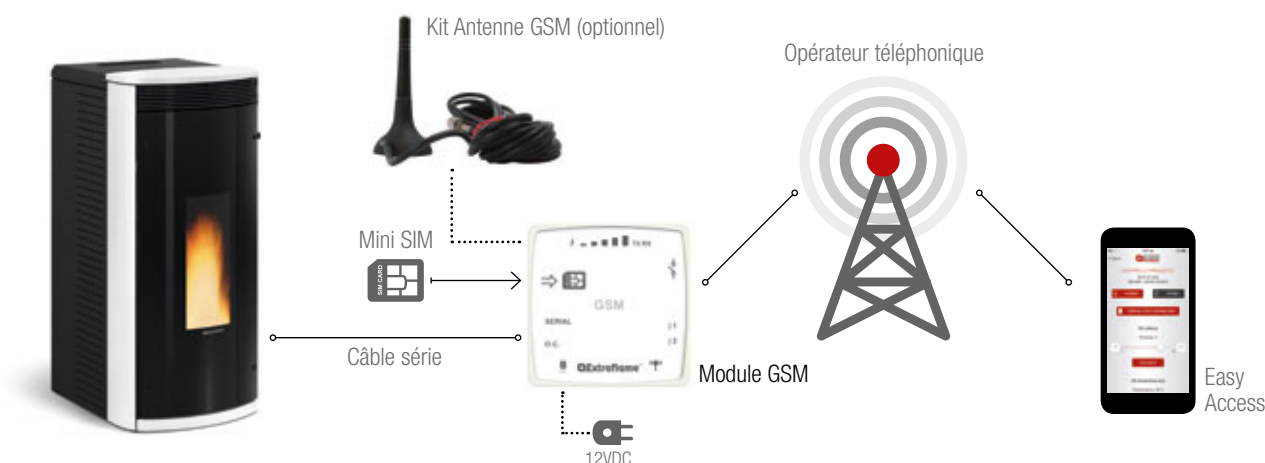
Schéma Module GSM
